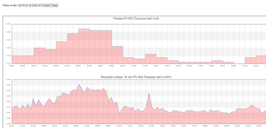
Slika 20: Monitoring porab in pretokov pitne vode na dnevem nivoju (Vir: Portal Petrol za dan 26.4.2023)
