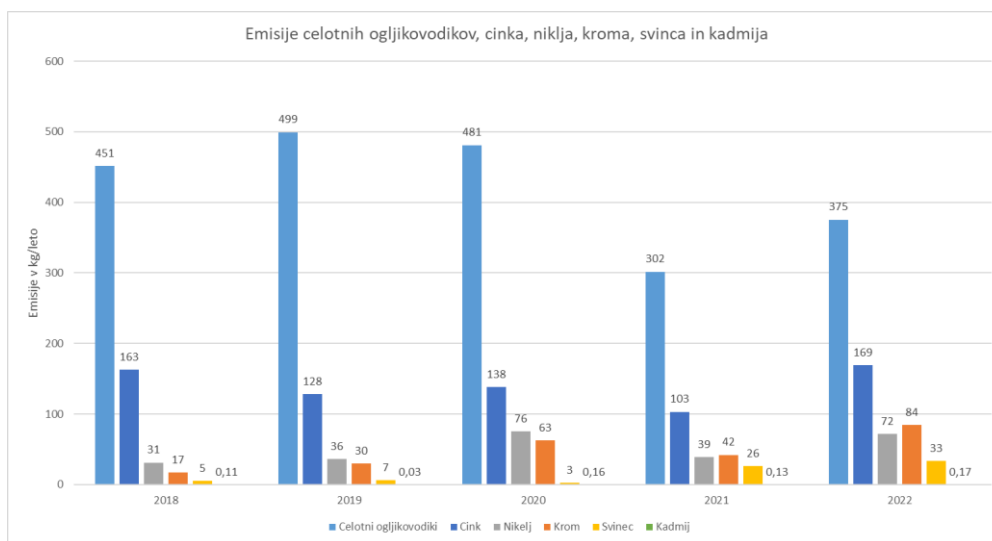
Slika 16: Emisije celotnih ogljikovodikov, cinka, niklja, kroma, svinca in kadmija (Vir: Poročilo o obratovalnem monitoringu odpadnih vod za podjetje SIJ Metal Ravne d.o.o., za leto 2022)
