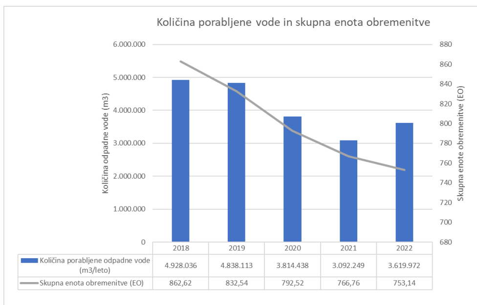
Slika 15: Količina porabljene vode in skupna enota obremenitve (Vir: Poročilo o obratovalnem monitoringu odpadnih vod za podjetje SIJ Metal Ravne d.o.o., za leto 2022)
